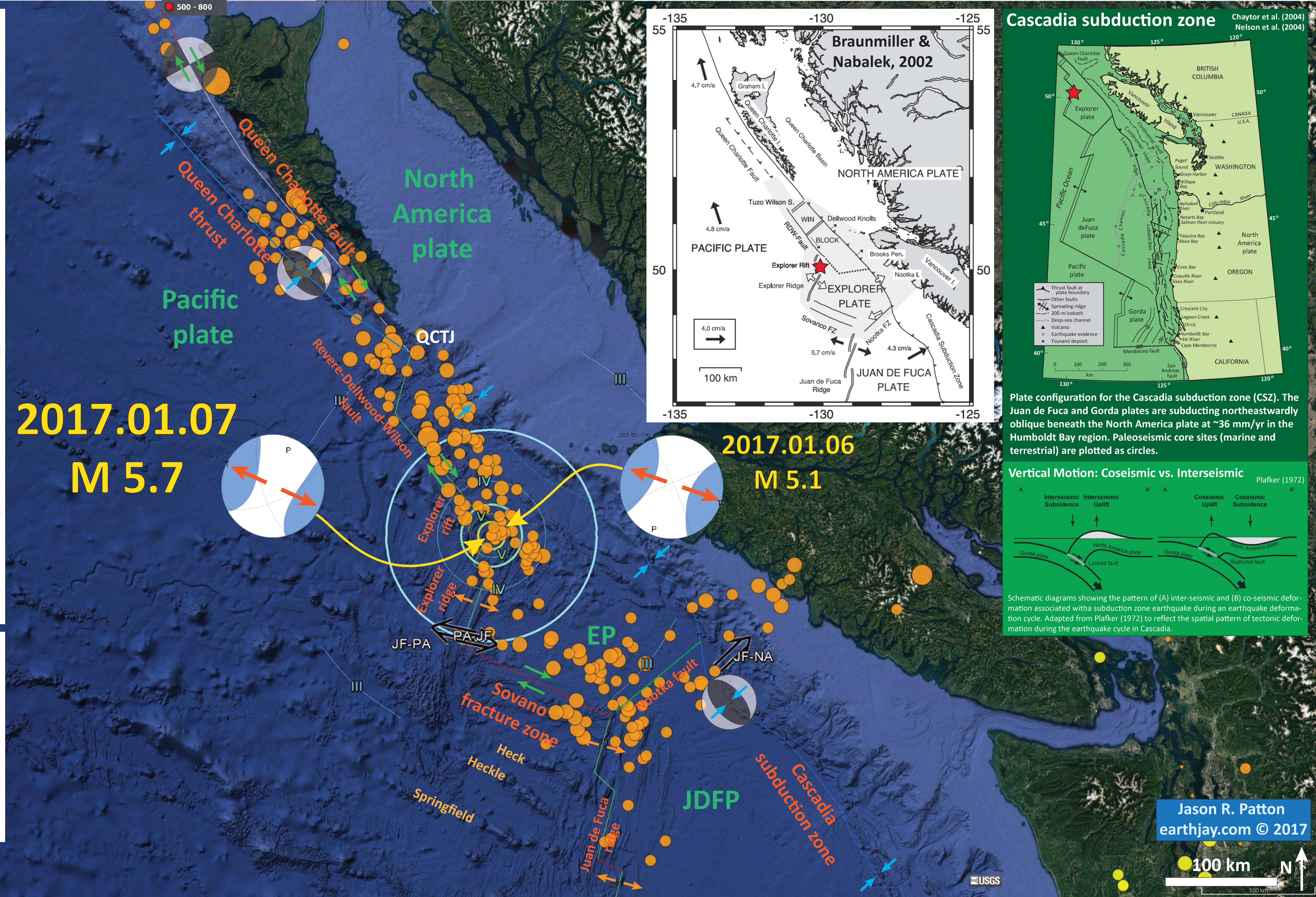
Braunmiller & Nabalek, 2002
