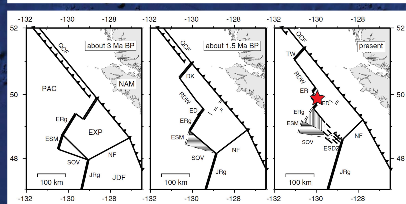
Braunmiller & Nabalek, 2002
