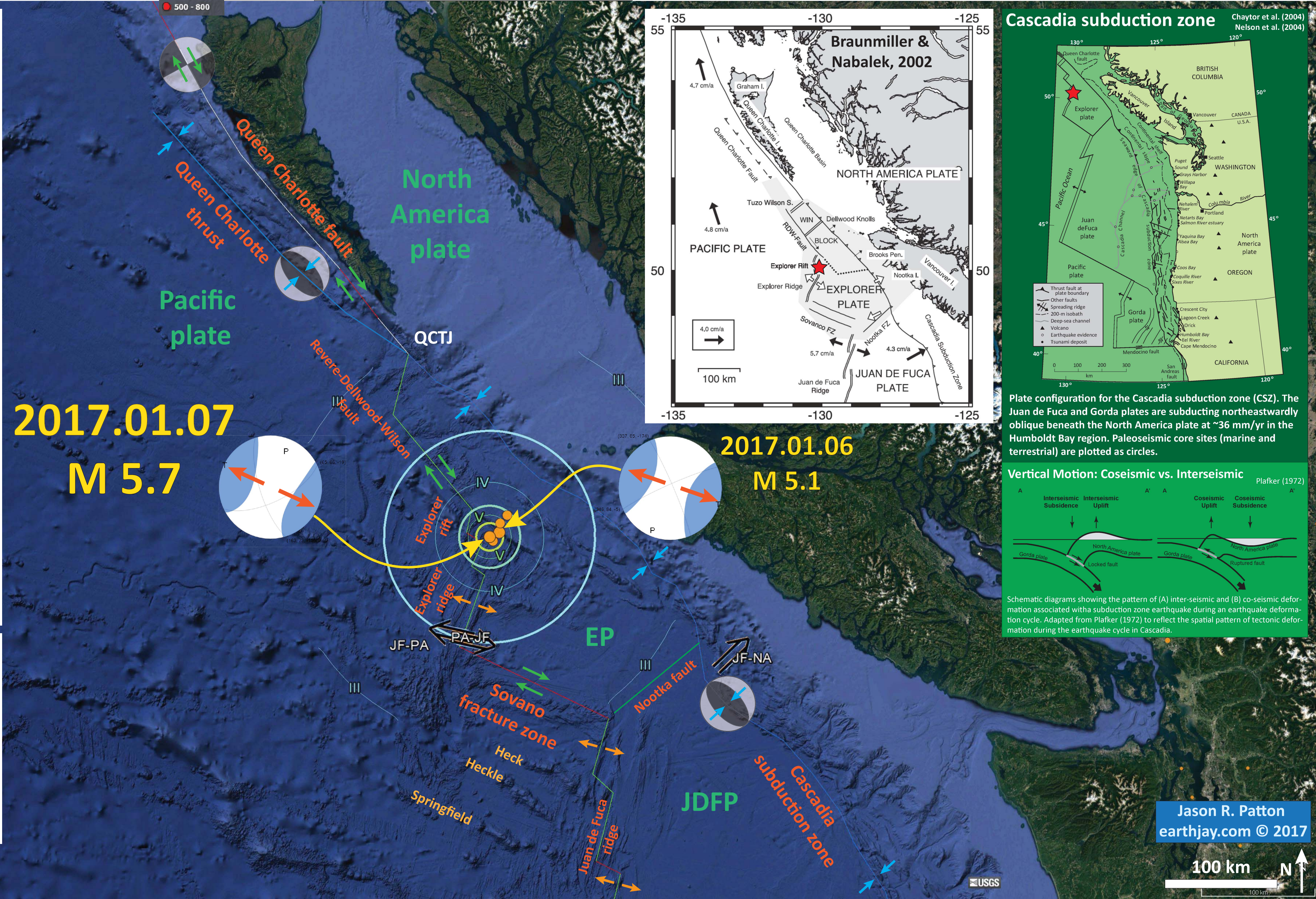
Braunmiller & Nabalek, 2002
