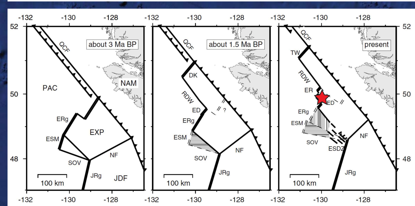
Braunmiller & Nabalek, 2002
